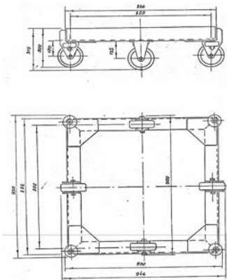
Рис.1. Тележка для транспортирования мусоросборников из мусороприемных камер грузоподъемностью 500 кг
