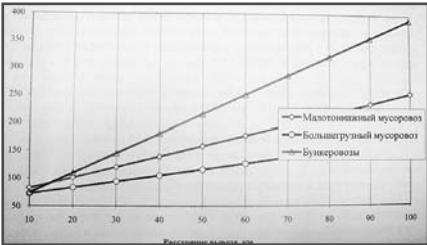
Рис. 2. Динамика роста себестоимости вывоза отходов для различных типов мусоровозов в зависимости от расстояния транспортирования
